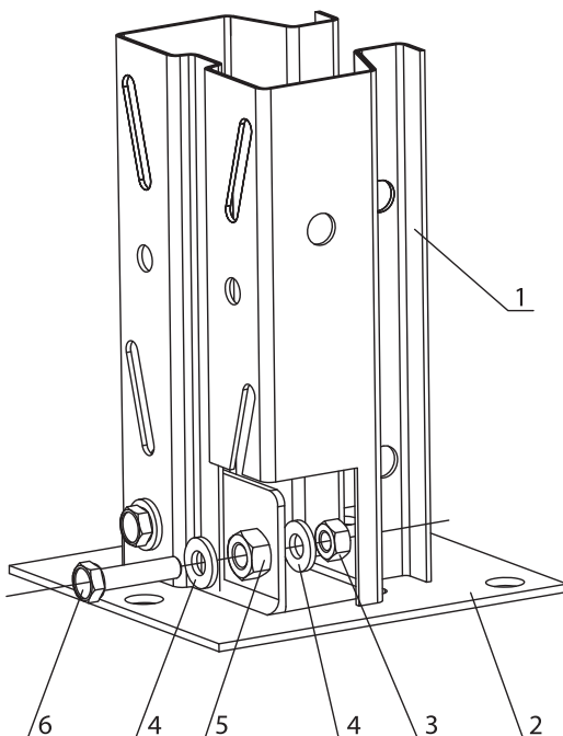
Рис 1. Установка подпятника на стойку.
